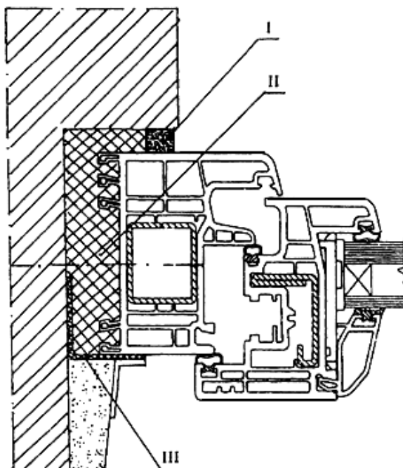
Рисунок 1 - Принципиальная схема монтажного шва
