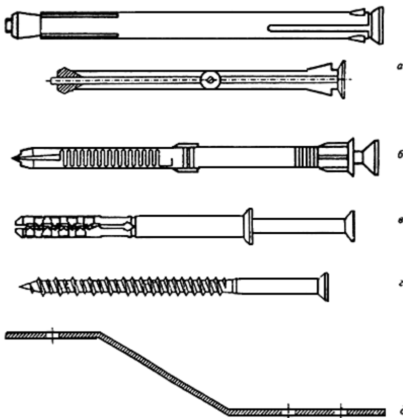
Рисунок Б.1 - Примеры крепежных элементов
