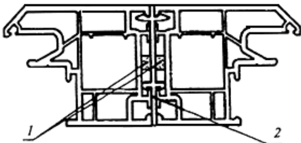
Рисунок А.15 - Узел соединения оконных коробок
