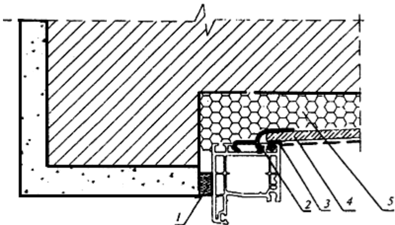
Рисунок А.13 - Узел бокового и верхнего примыкания оконного блока к проему стены с четвертью и отделкой внутреннего откоса панелями
