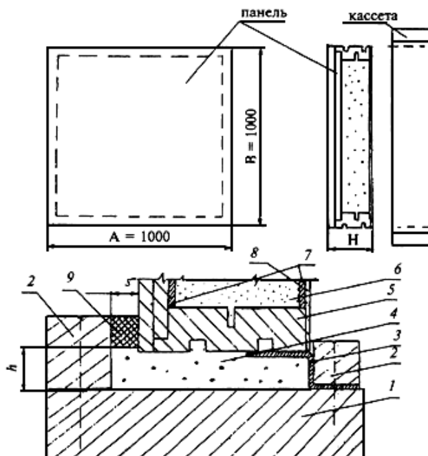
Рисунок 3 - Устройство для испытаний монтажных швов на воздухо-, водопроницаемость и звукоизоляцию
