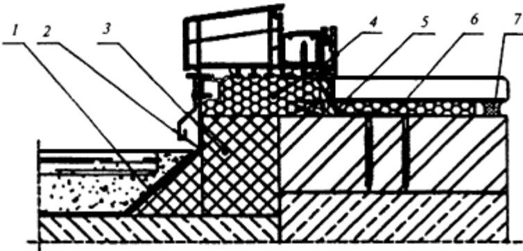
Рисунок А.11 - Монтажный шов в нижнем узле примыкания коробки балконной двери
