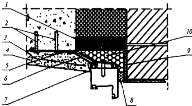
Рисунок А.5 - Узел верхнего примыкания оконного блока к перемычке из стального уголка в проеме многослойной стены с облицовкой кирпичом
