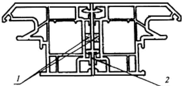
Рисунок А.15 - Узел соединения оконных коробок
